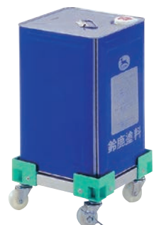
一斗缶台車 S型 1缶用 ●¥11,500 252(246)×252(246)×125(105) キャスター:φ50(ナイロン、自在車4ヶ、S2ヶ付) ジョイント色:グレー
