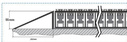
断面図 スロープの高さは55mm
