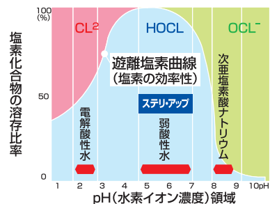
塩素の各pH領域における化学変化による溶存比率
